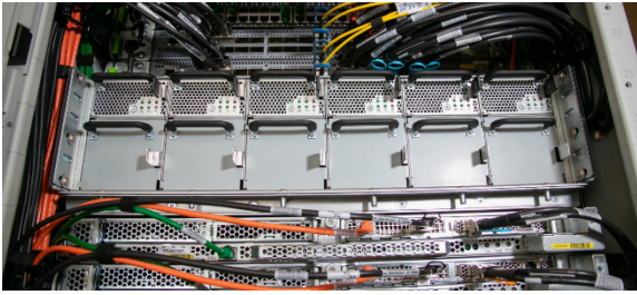
Figura 3 - AWS Outposts AC-to-DC alimentatori e distribuzione dell'alimentazione tramite sbarra
