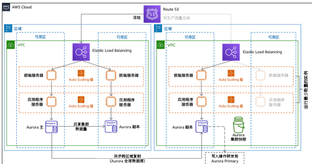
图 21：热备用架构
